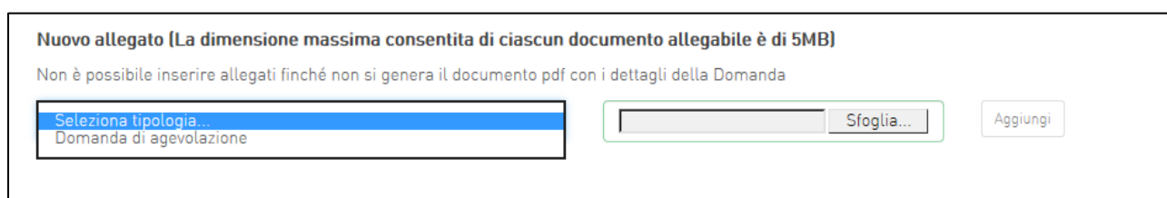
Figura 45 – Caricamento domanda
